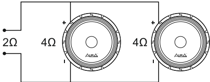
Параллельное подключение
