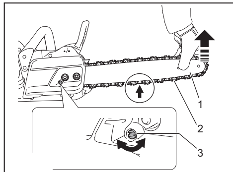
► 1. Пильная шина 2. Пильная цепь 3. Винт регулировки цепи
