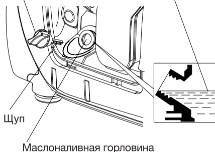
Маслоналивная горловина
