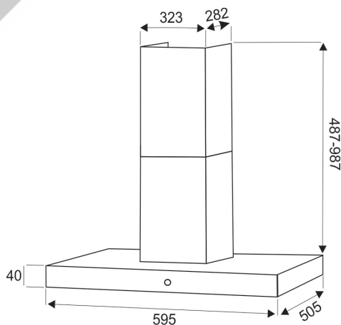
Рис. 1 Внешний вид кухонной вытяжки и схема размеров
