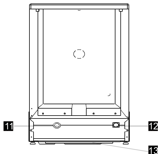
Вид сзади
