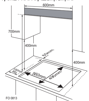
СОРҒЫШЫ БАР ПІСІРУ ПАНЕЛІН ОРНАЛАСТЫРУҒА ҚАЖЕТТІ АРАҚАШЫҚТЫҚТАР
