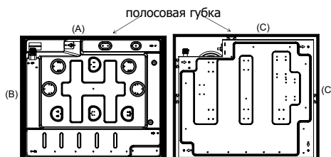
вид поддона
