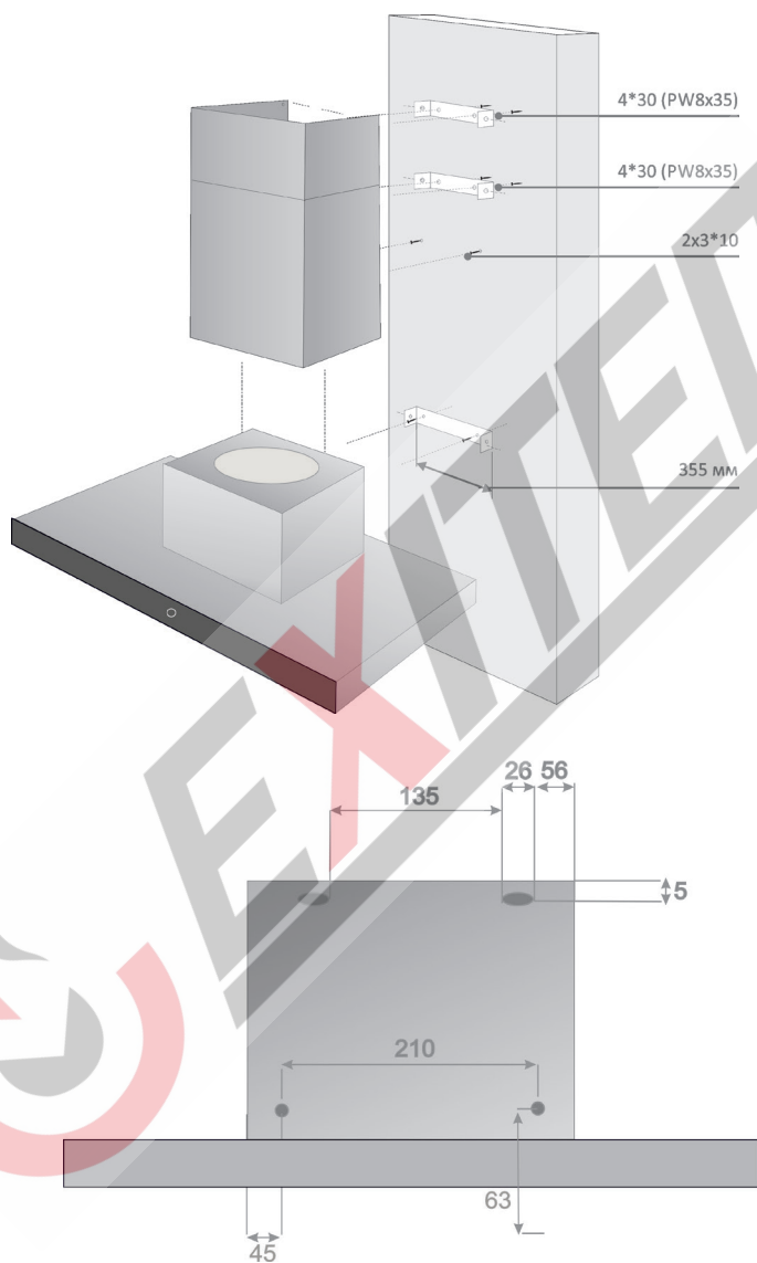
Рис. 8 Схема монтажа вытяжки
