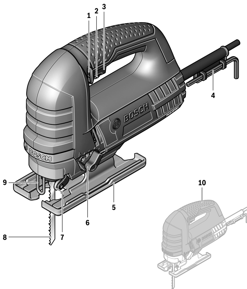
GST 8000 E
