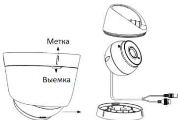
Рисунок 2-11 Демонтаж камеры
