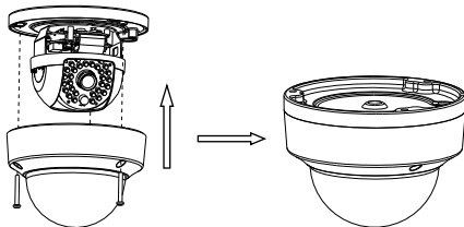
Рисунок 2-9 Установка купола
