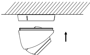
Рисунок 2-13 Установка камеры на платформу
